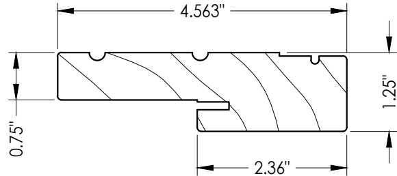
19 20 HEAD & SIDE JAMB
